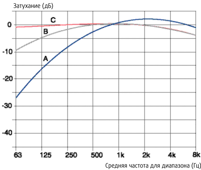
Рис. 7. Выравнивание с А-, В- или С-фильтрами
