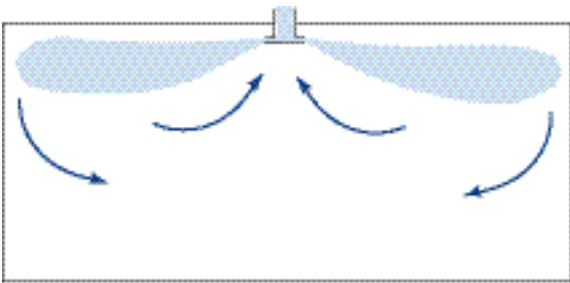
Рис. 21. Горизонтальная подача воздуха потолочным диффузором
