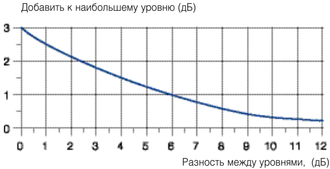
Рис. 5. Логарифмическое сложение
