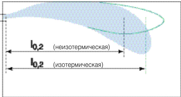
Рис. 23. Разница между длиной изотермической и неизотермической струй.
