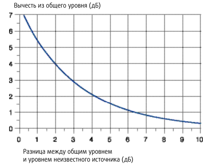
Рис. 6. Логарифмическое вычитание
