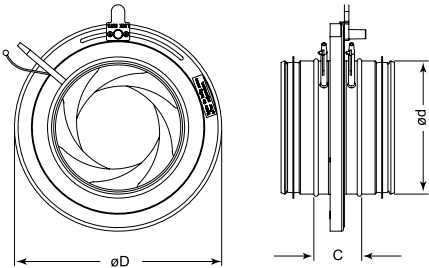
Einstecktiefe beidseitig 35 mm
