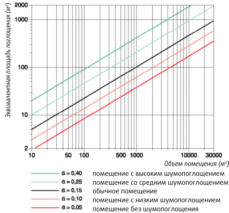
Рис. 2. Оценка эквивалентной площади поглощения
