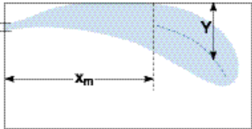
Рис. 13. Точка отрыва воздушной струи (Xm) и отклонение (Y)
