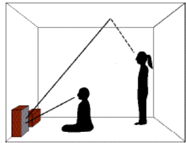
Рис. 4. Прямой и отраженный звук.
