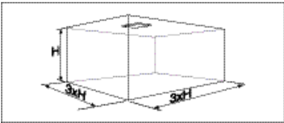
Рис. 18. Небольшое помещение, вентилируемое одним потолочным диффузором Если помещение
