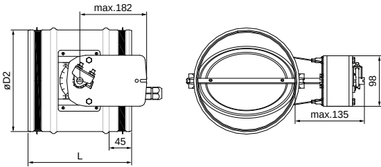
TUNE-R-M с автоматическим управлением
